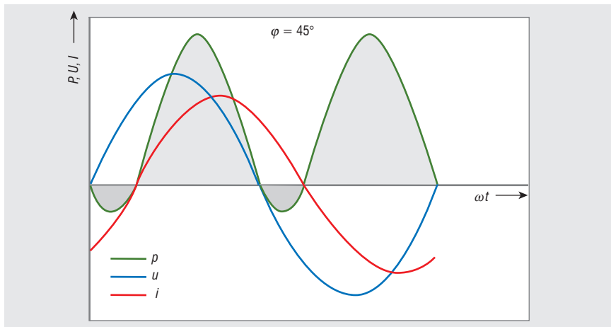
Bild 2: Spannung, Strom und Leistung bei ohmsch/induktiver Last ( \varphi = 45^\circ )
