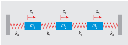
Bild 2: Eindimensionales Modell einer eingespannten Welle
